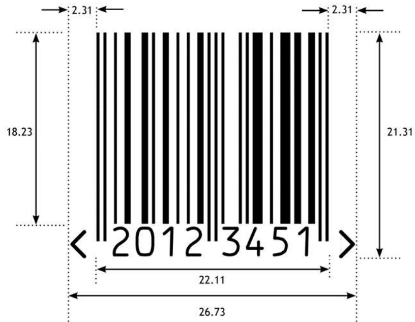
Abbildung 5.2.6.6-4. UPC-E Strichcode
