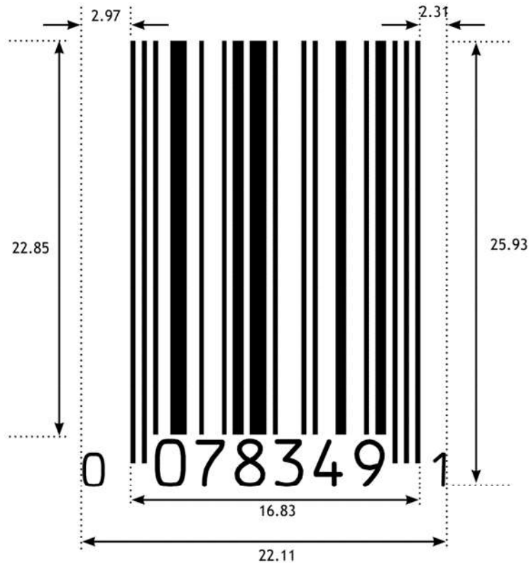
Abbildung 5.2.6.6-4. UPC-E Strichcode
