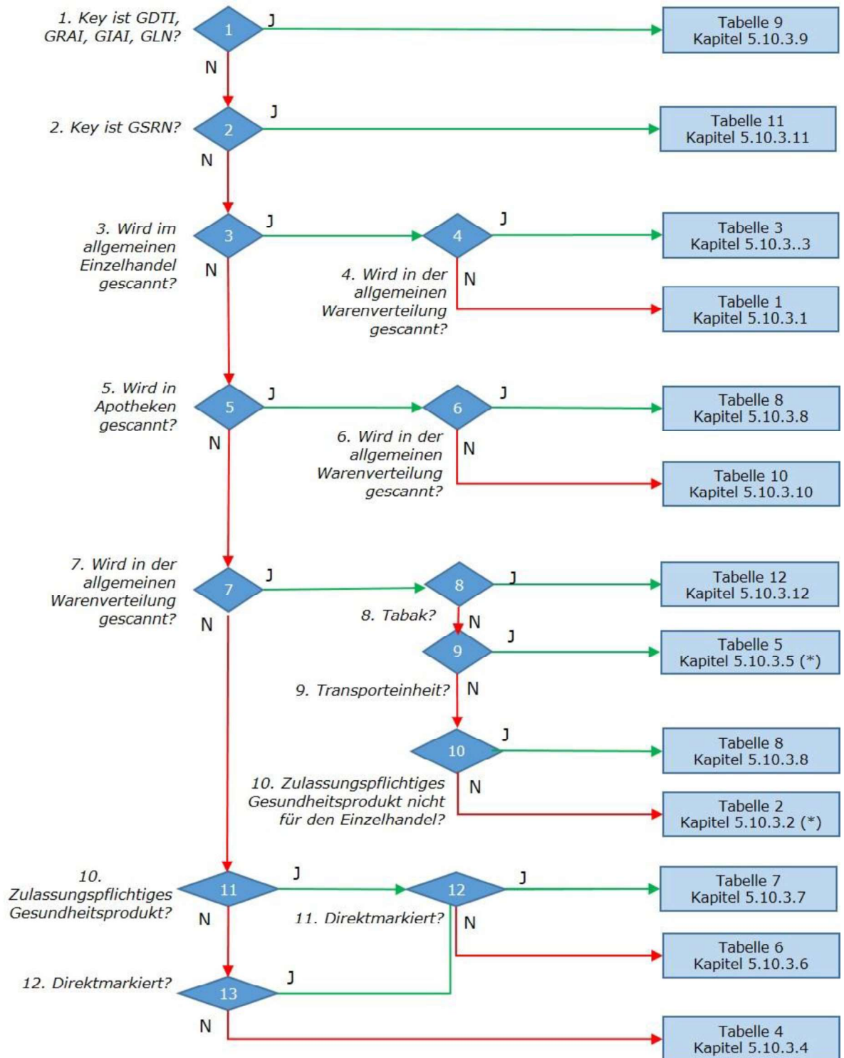
Abbildung 5.12.2.6-2. Entscheidungsbaum
