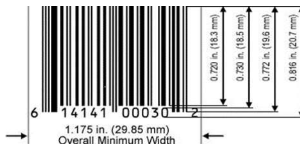
Abbildung 5.12.6.3-1. EAN/UPC Symbol angegeben mit der minimalen Höhe und der Gesamtbreite für eine Vergrößerung von 75% bis 80%
