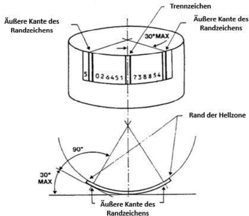
Abbildung 6.2.3.2-2. Zusammenhang zwischen Symbol und Wölbung
