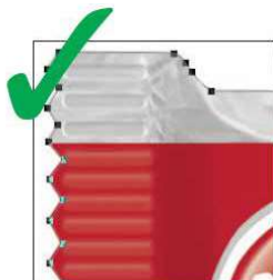
Beschneidungspfad optimal
