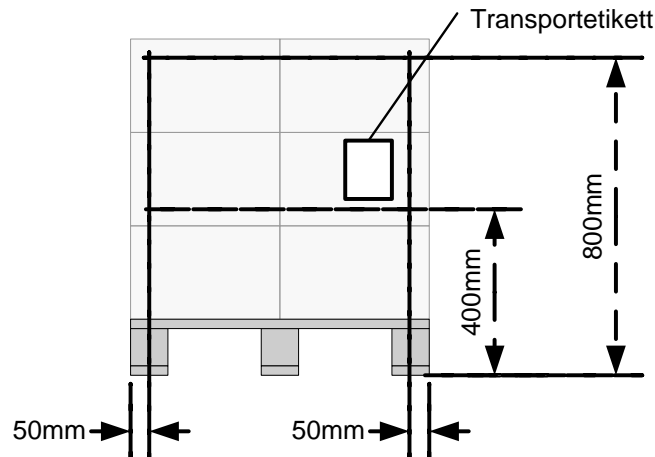
Abbildung: Transportetikettenposition
