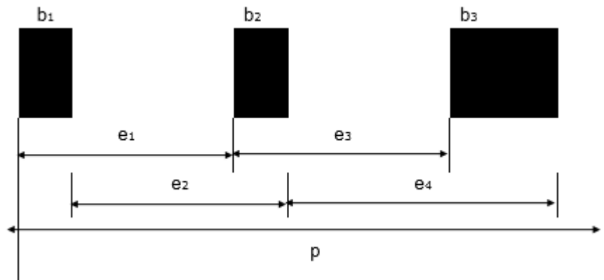
Abbildung 5.4.5-1. Breitenmaße
