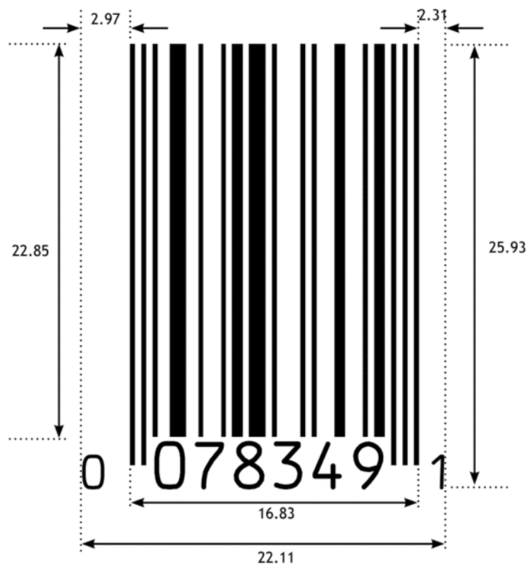
Abbildung 5.2.6.6-4. UPC-E Strichcode
