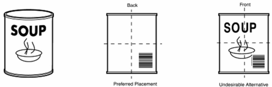
Abbildung 6.4.5-1. Barcodeplatzierung auf Dosen und Zylindern
