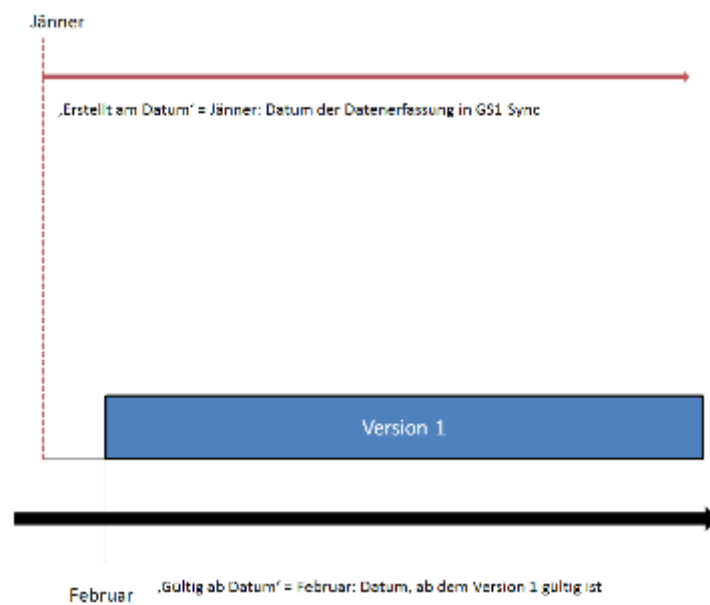
Abbildung 5: Versionierung - Version 1
