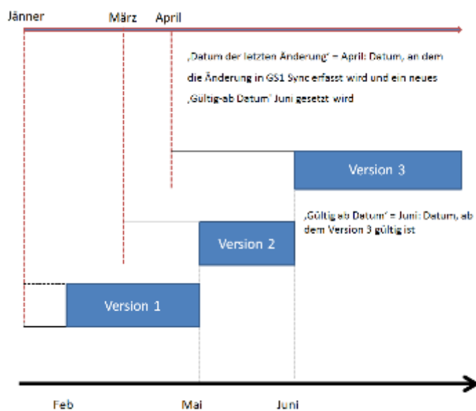
Abbildung 7: Versionierung - Version 3
