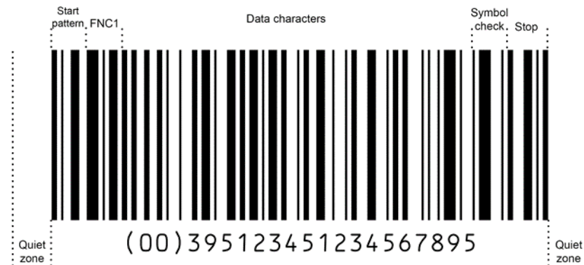
Abbildung 5-34 Allgemeines Format eines GS1-128 Strichcodes
