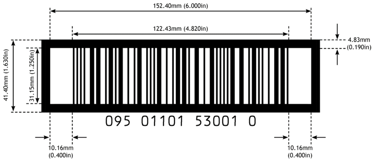
Abbildung 5-33 ITF-14 Symbol: Abmessungen bei einer X-Modulbreite von 1,016 mm (Nominalgröße) (0.040 in.)
