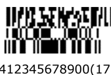
Abbildung 5-63 GS1 DataBar Stacked Symbol mit einer 2-spaltigen CC-A Komponente
