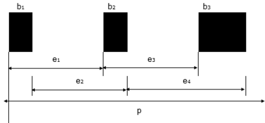
Abbildung 5-38 Breitenmaße
