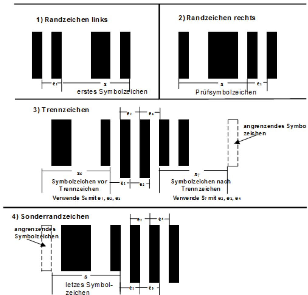
Abbildung 5-22 Messgrößen für EAN/UPC Hilfszeichen
